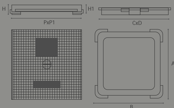
>> HIDRAULICA B-125
